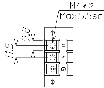
出力端子台詳細
