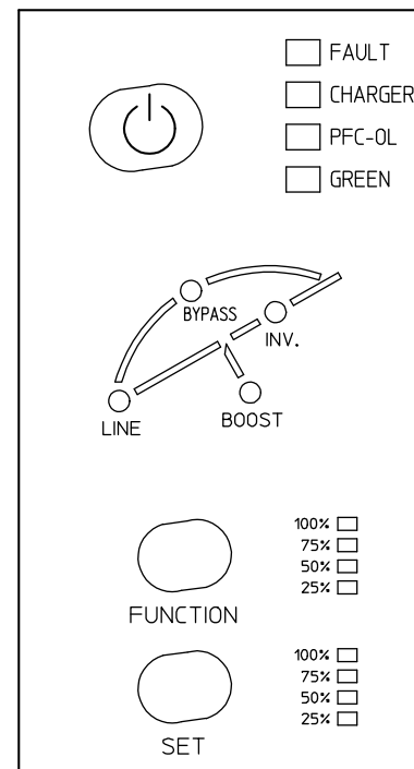
操作パネル詳細
