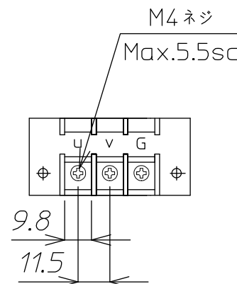
出力端子台詳細
