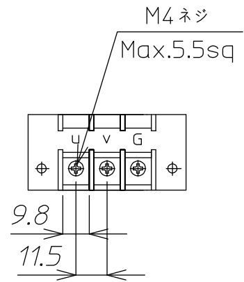
出力端子台詳細
