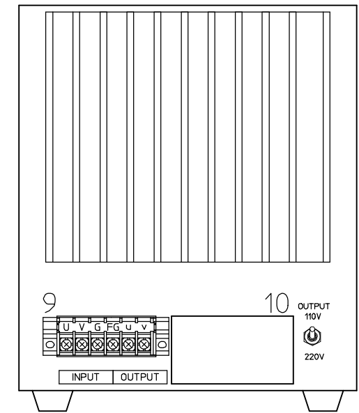
後面
