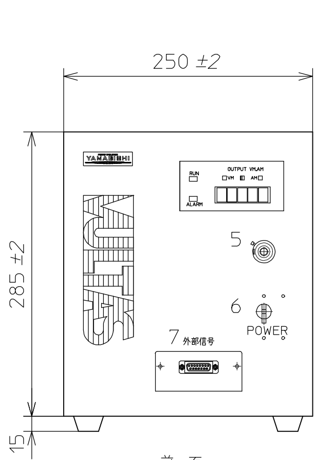
前面
