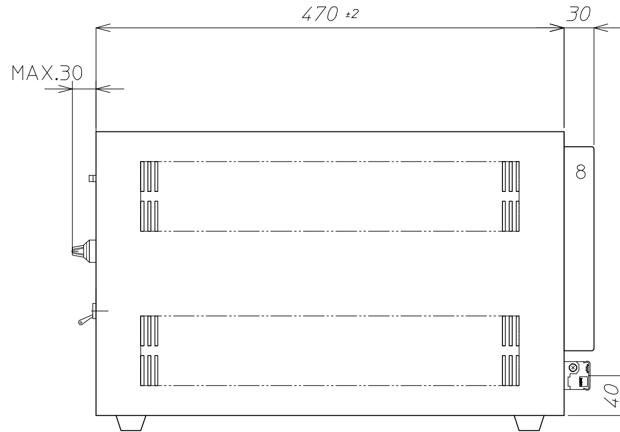
右側面
