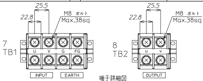
端子詳細図
