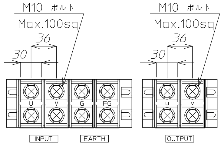
端子詳細図
