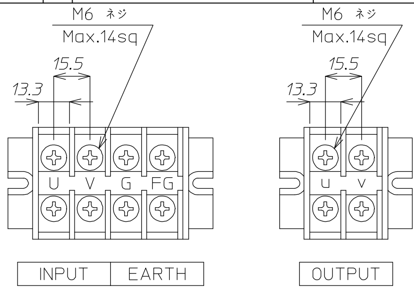
端子詳細図
