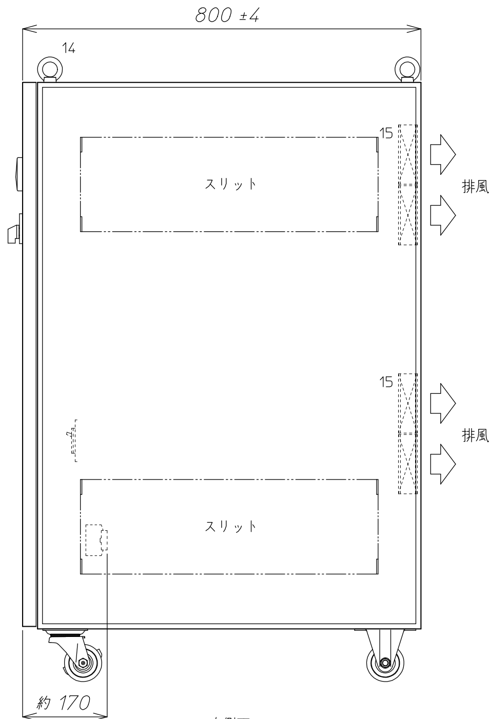
右側面
