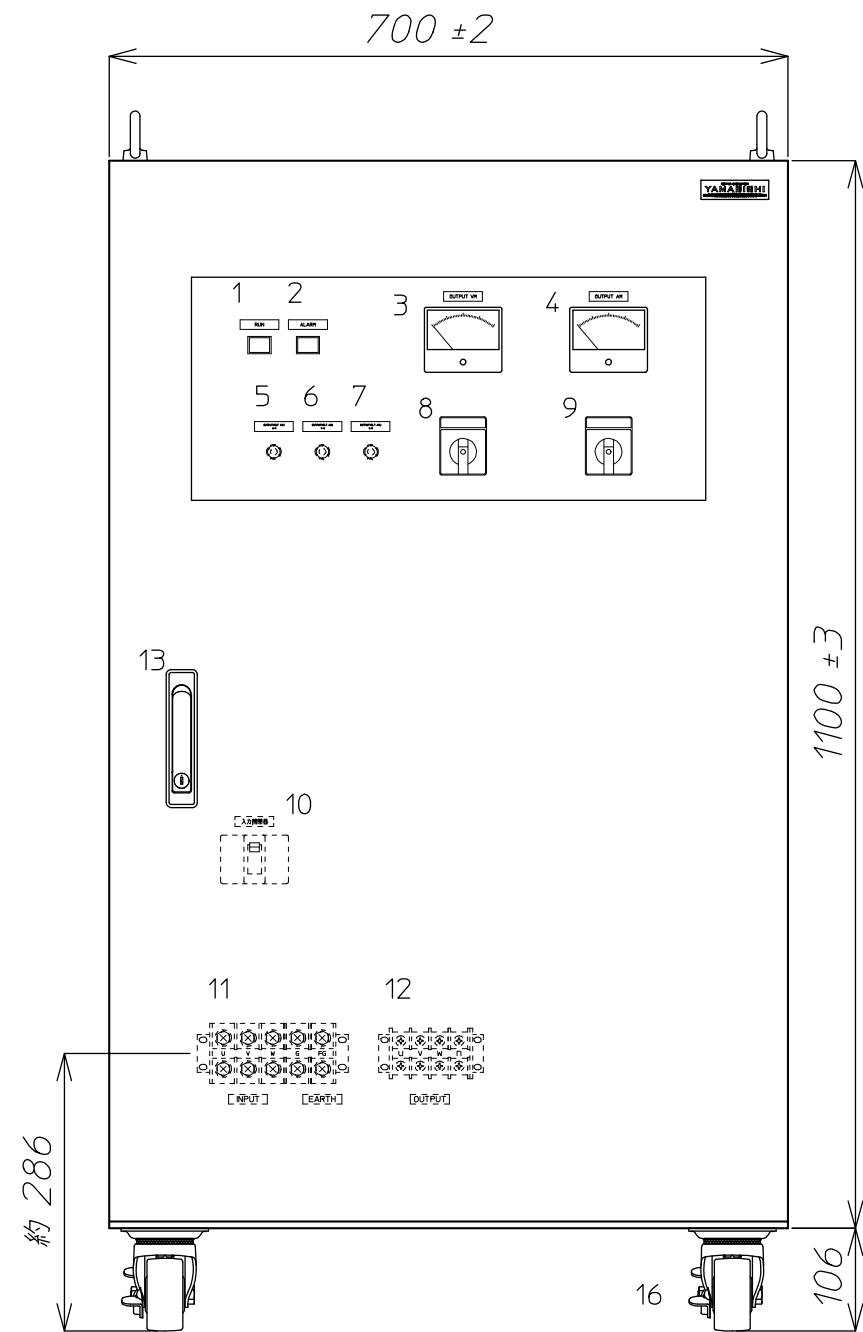
正面
