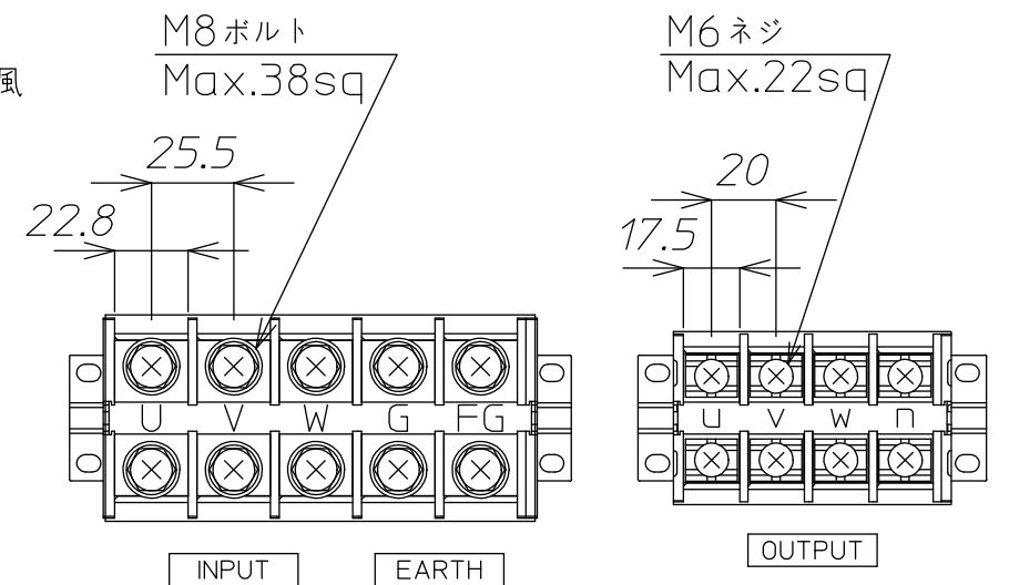
端子詳細図
