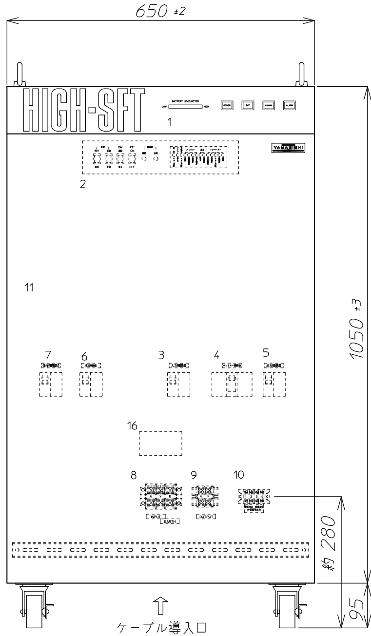
正面
