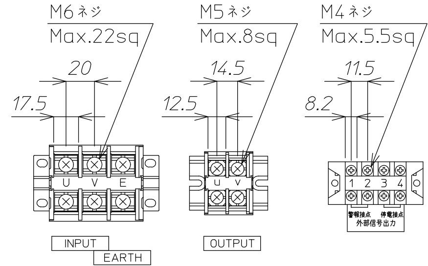
端子詳細図
