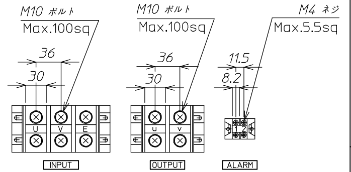
端子台詳細
