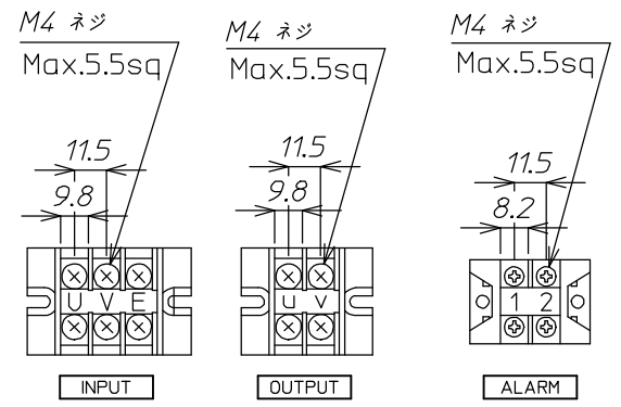
端子台詳細
