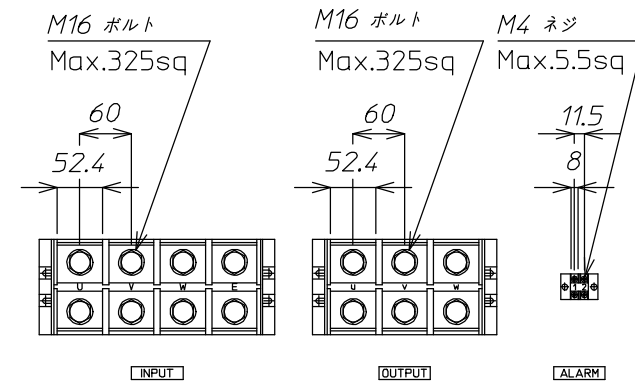
端子台詳細
