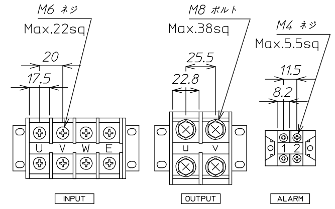
端子台詳細
