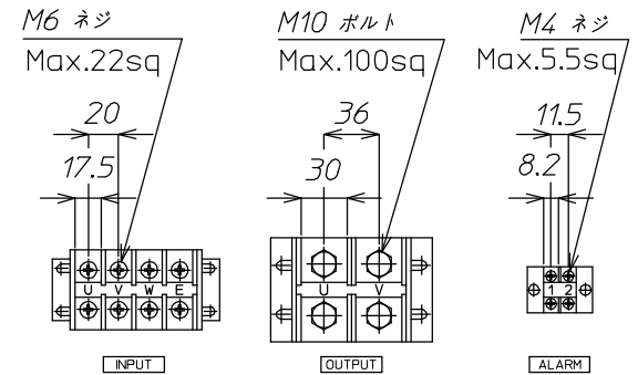
端子台詳細
