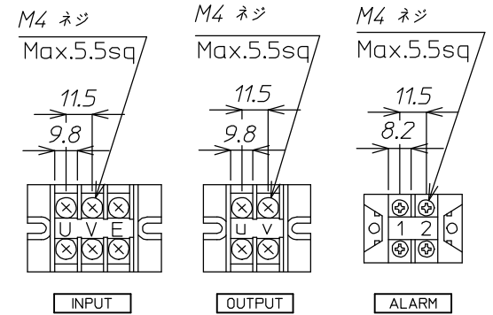
端子台詳細
