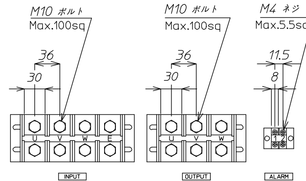
端子台詳細
