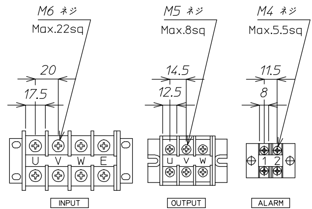
端子台詳細
