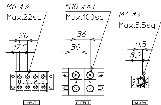
端子台詳細
