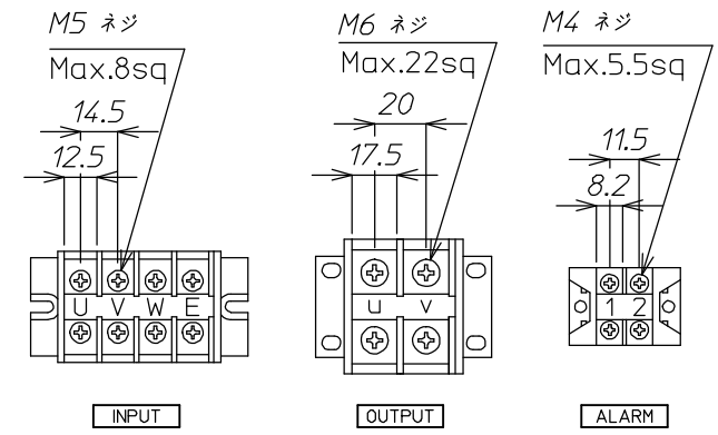
端子台詳細
