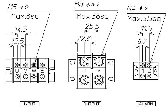
端子台詳細図
