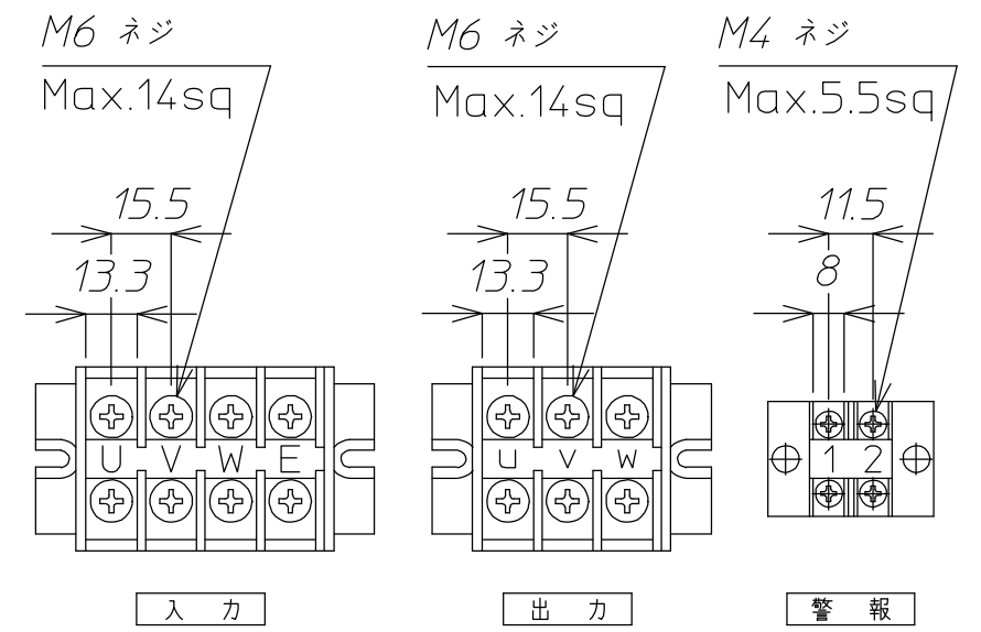
端子台詳細
