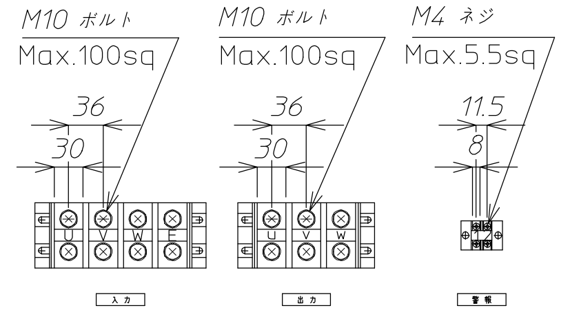
端子台詳細
