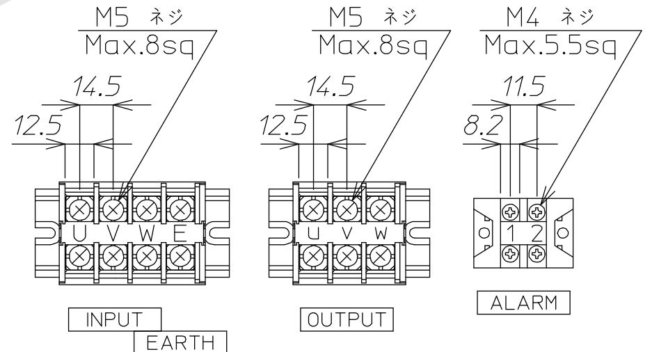
端子詳細図
