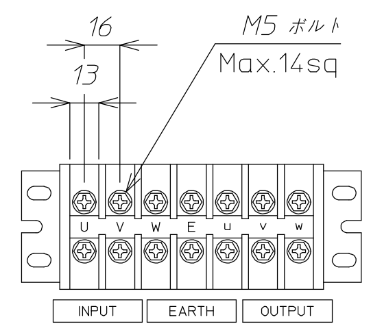
端子配置図
