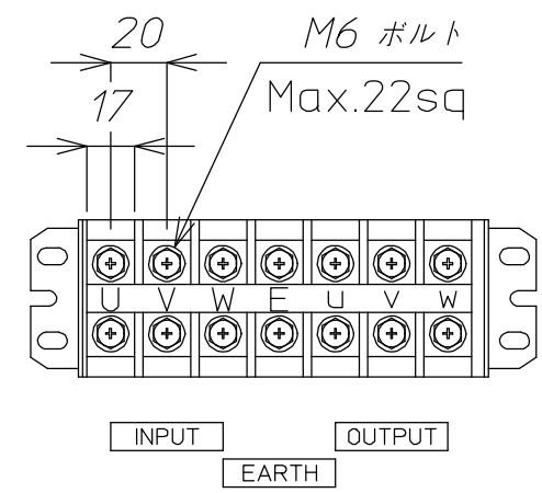
端子配列図
