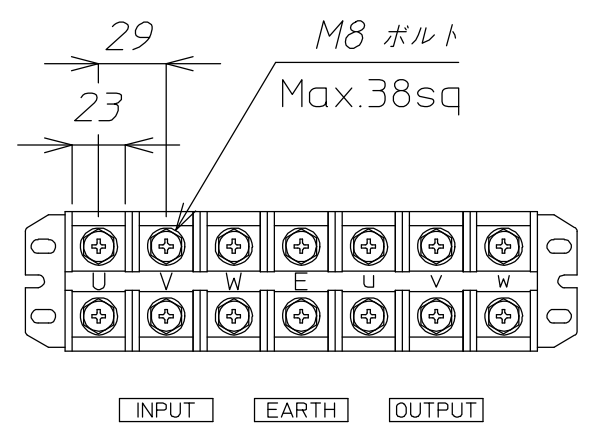
端子配置図
