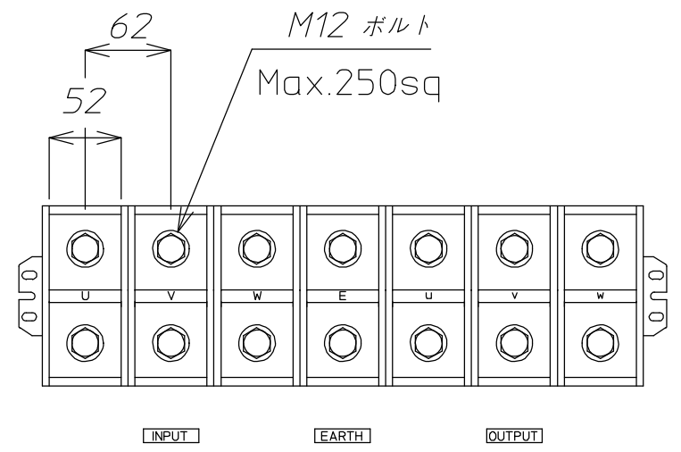
端子配置図
