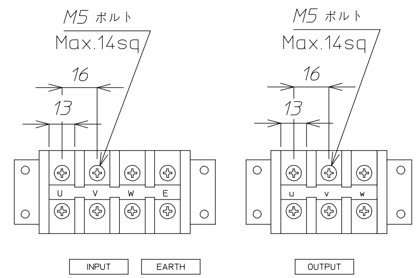
端子配置図
