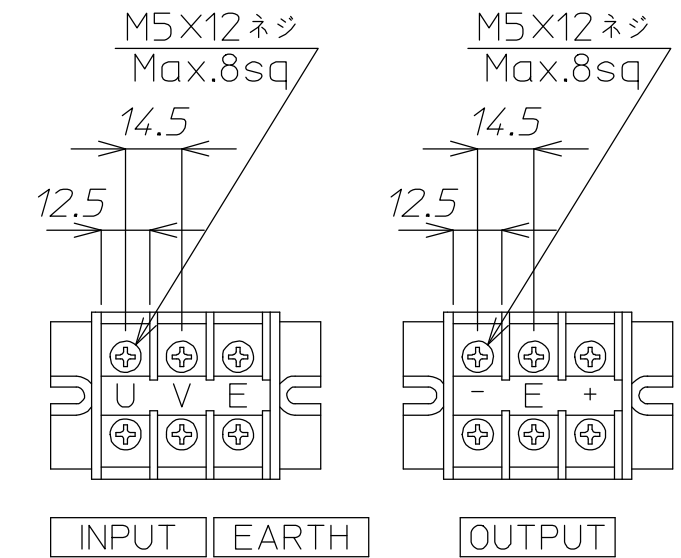
端子詳細図
