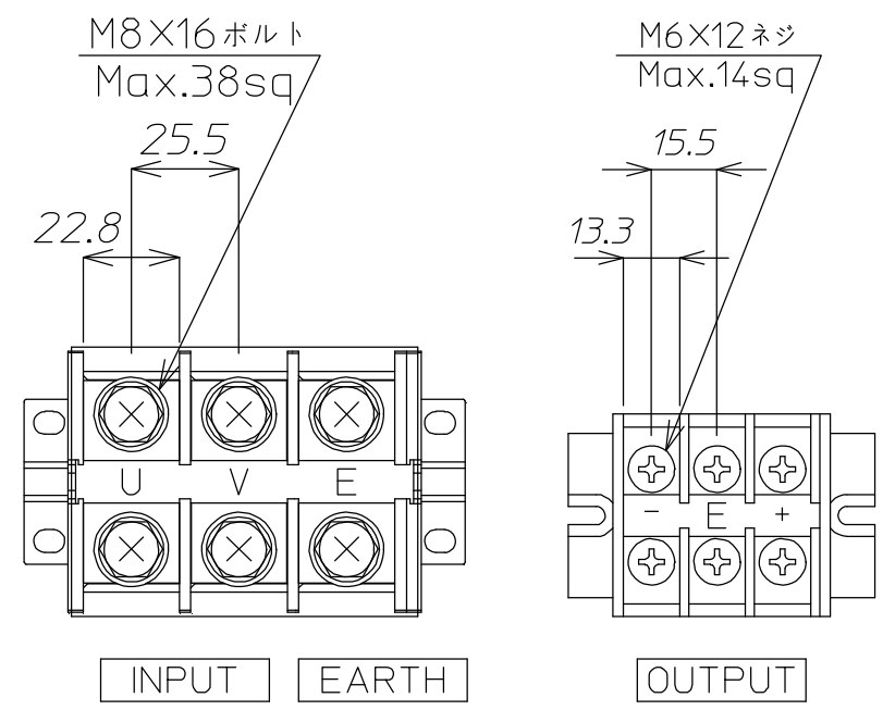
端子詳細図
