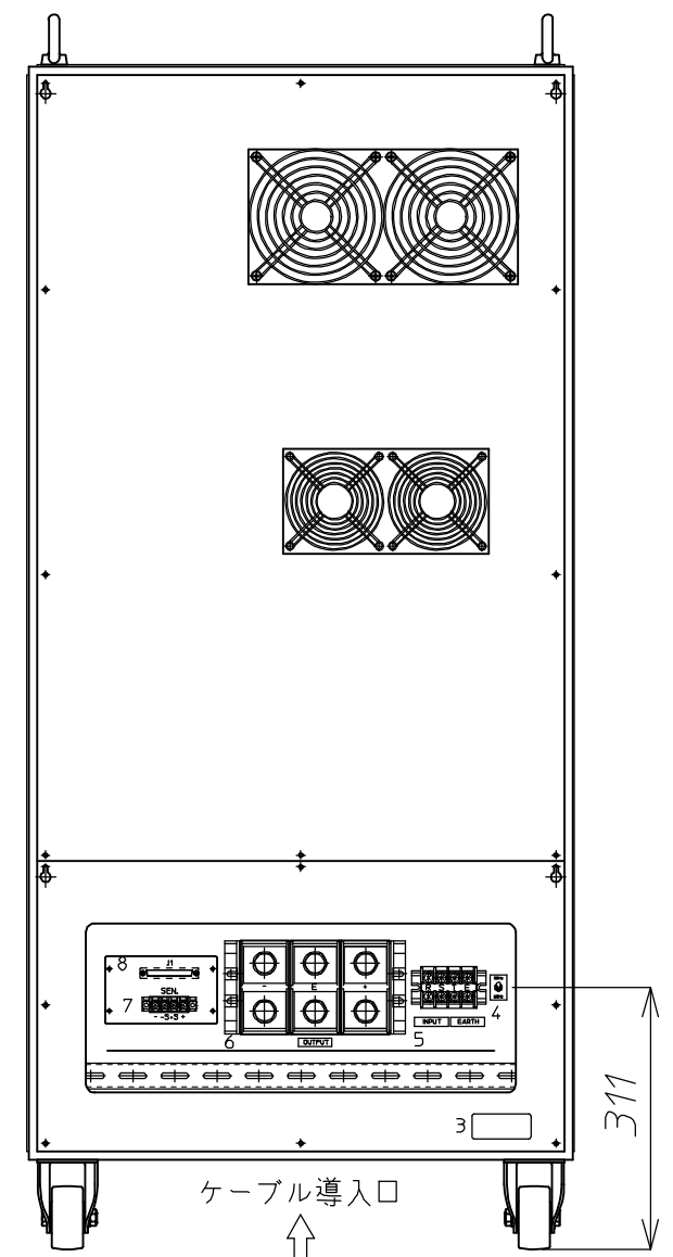
背面図
