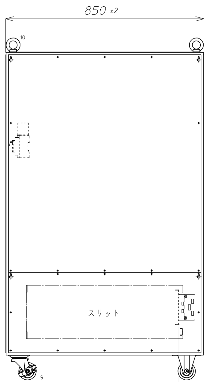
右側面図
