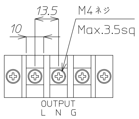
出力端子詳細図
