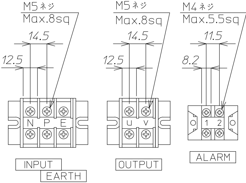
端子詳細図
