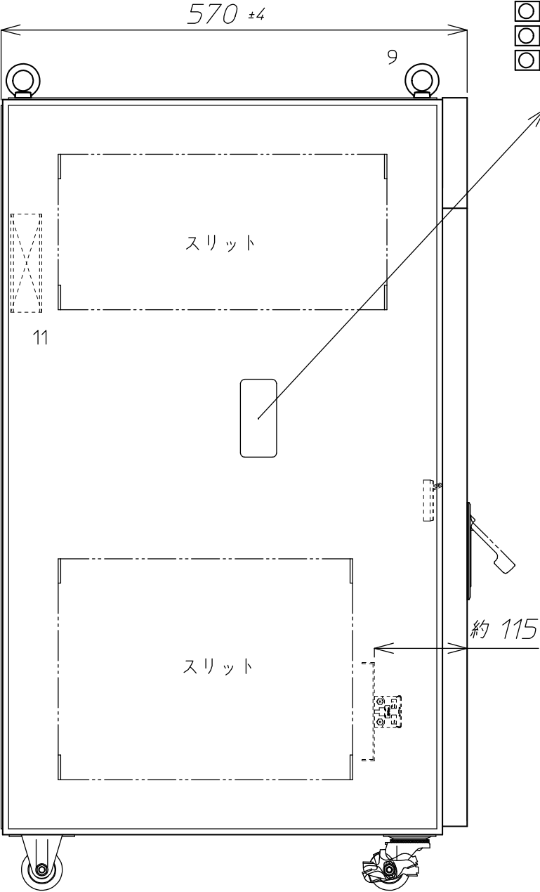
警報詳細図
