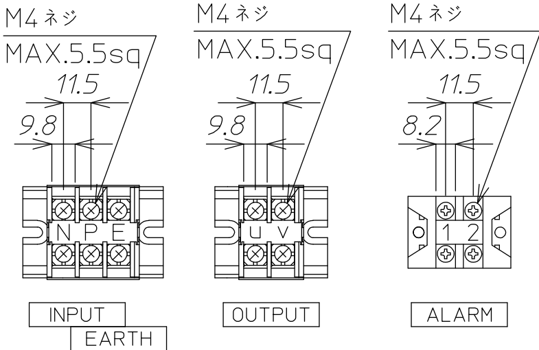
端子詳細図
