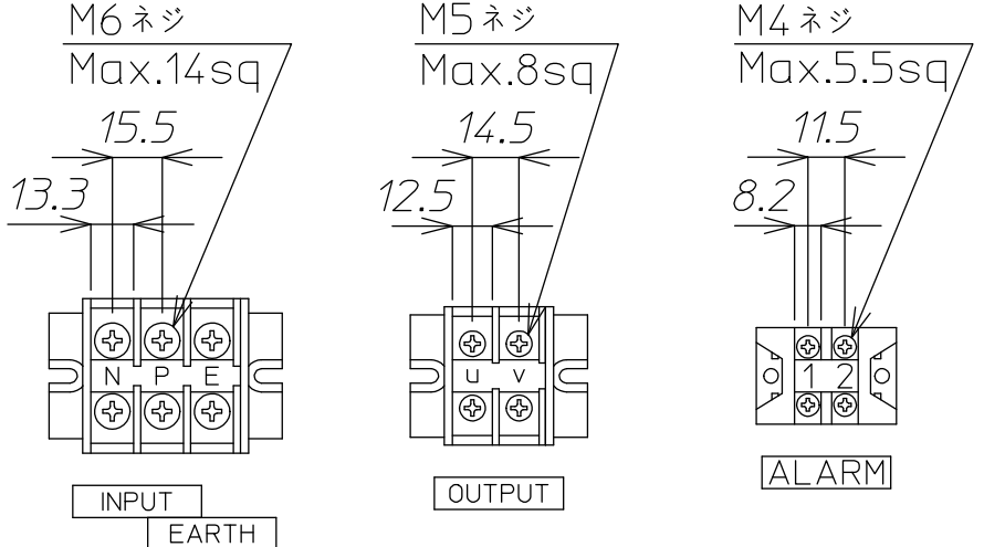
端子詳細図
