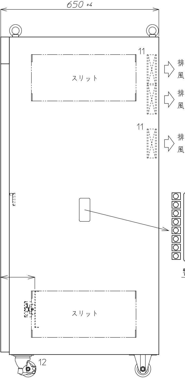
右側面図
