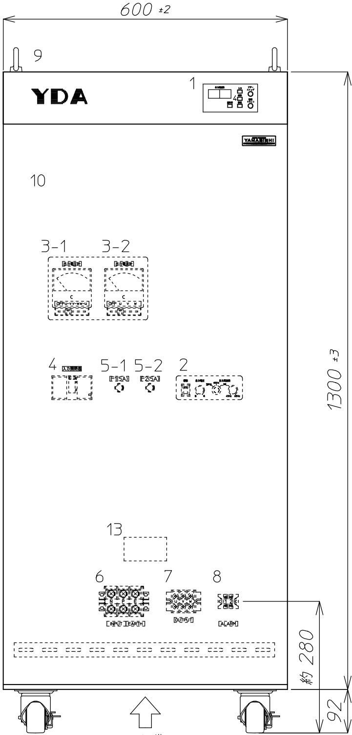
正面図
