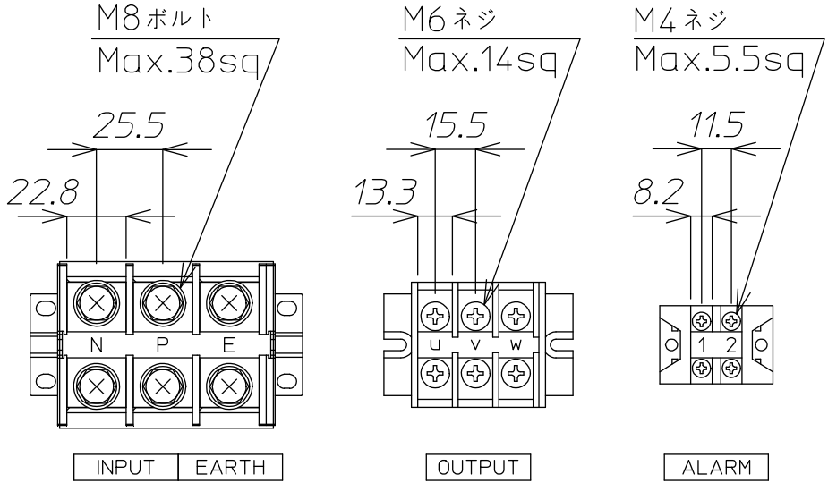
端子詳細図
