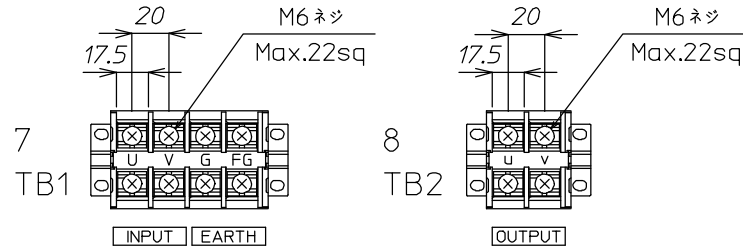
端子詳細図
