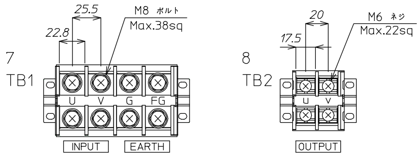
端子詳細図
