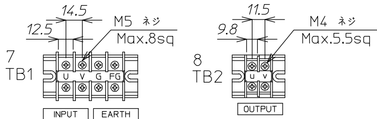
端子詳細図
