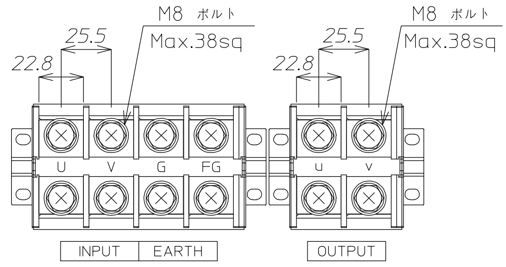
端子詳細図
