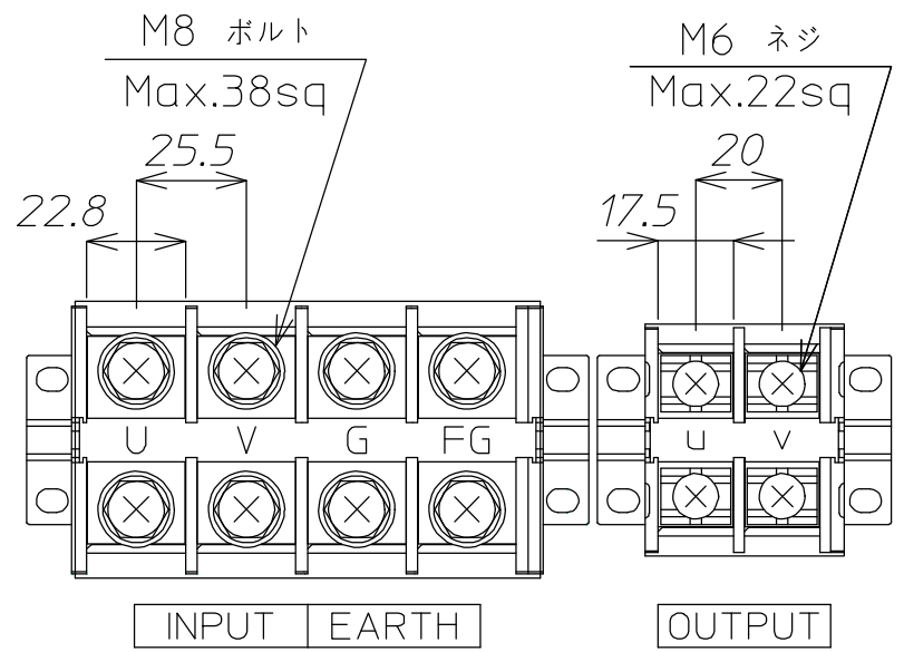
端子詳細図
