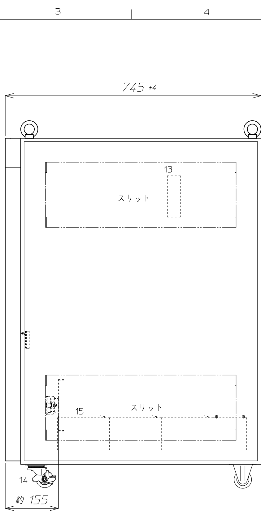
右側面
