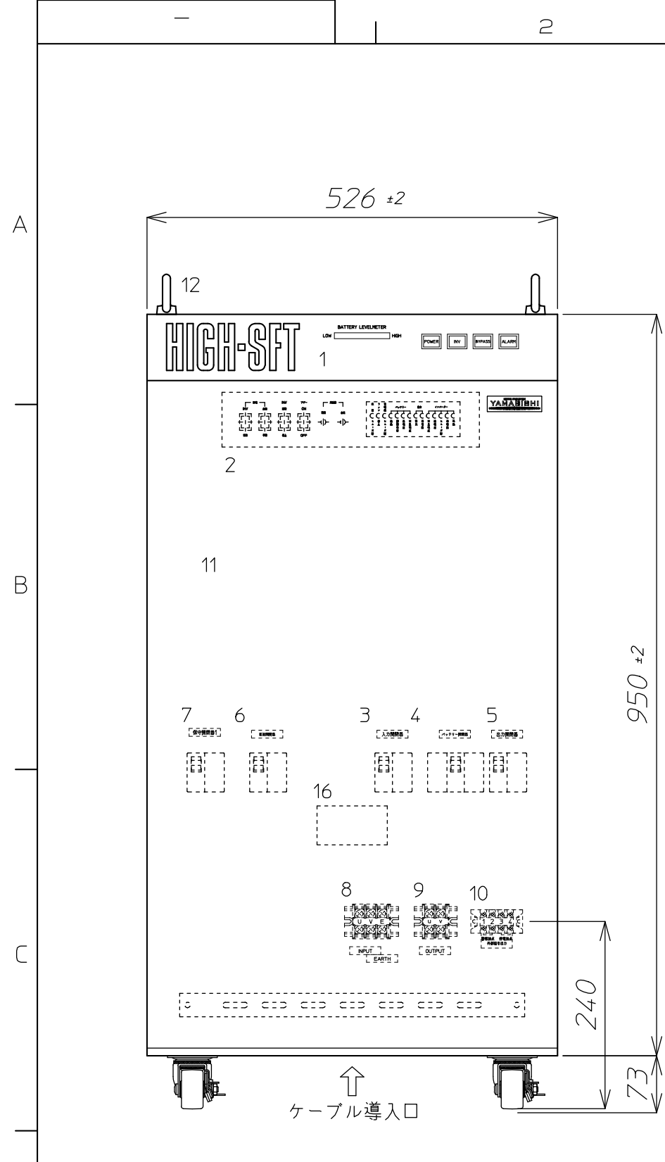
正面
