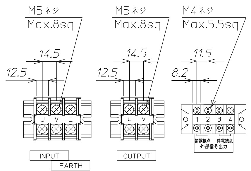
端子詳細図
