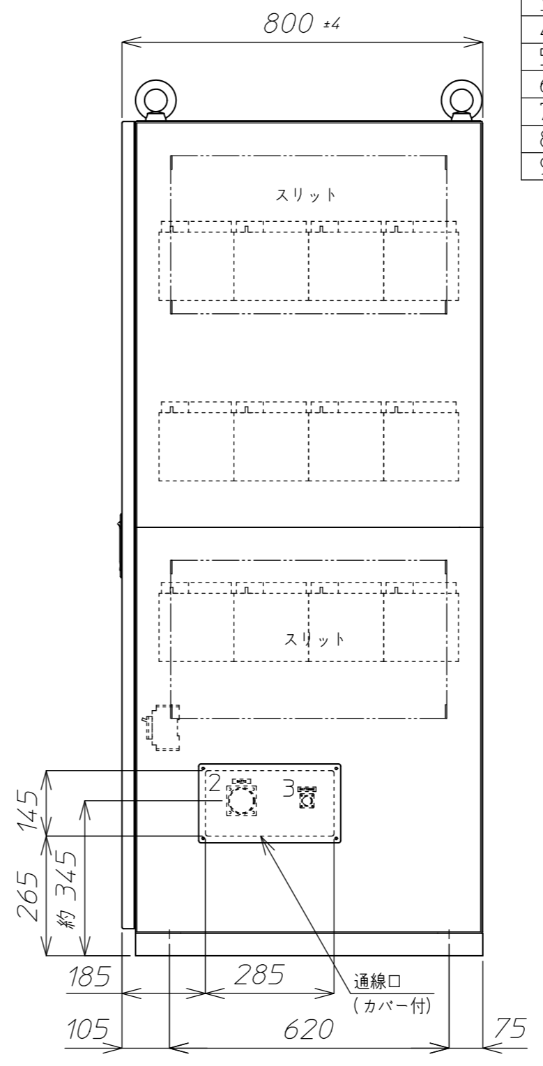
右側面
