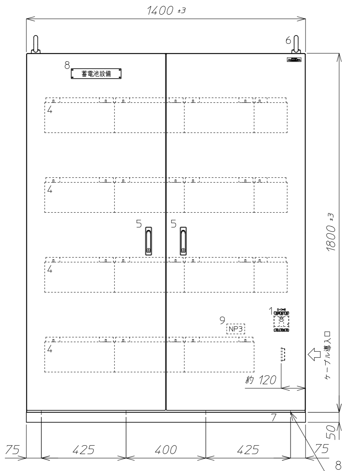
正面
