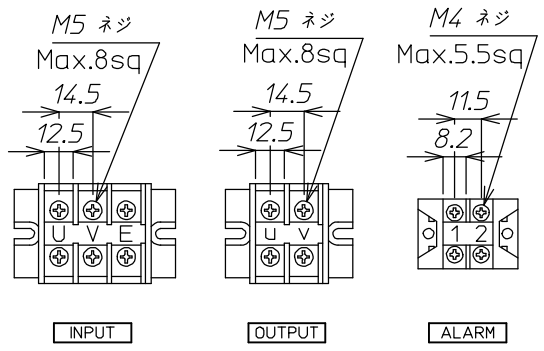
端子台詳細
