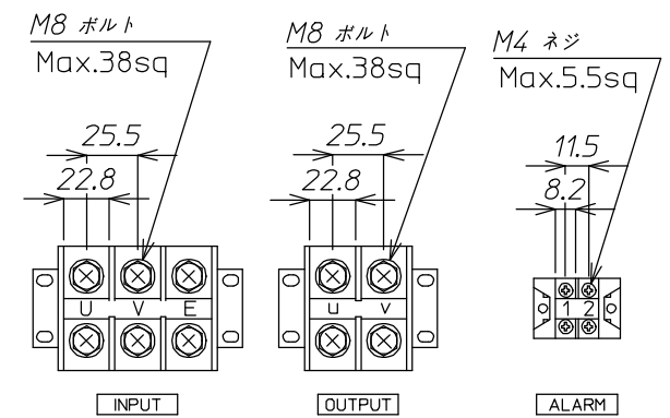
端子台詳細図
