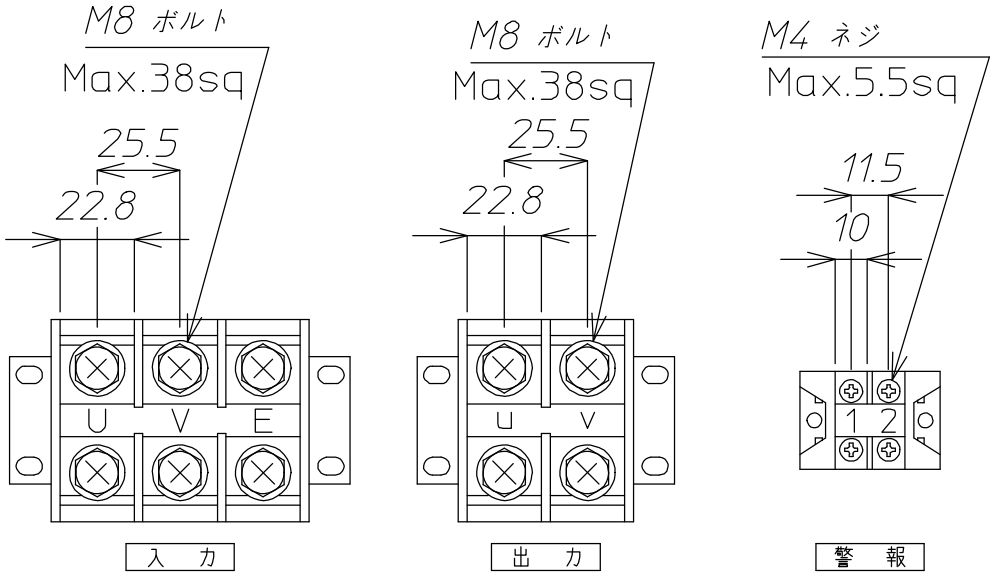
端子台詳細
