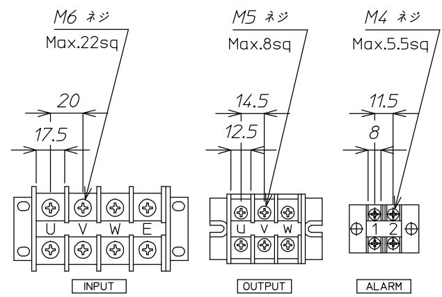
端子台詳細
