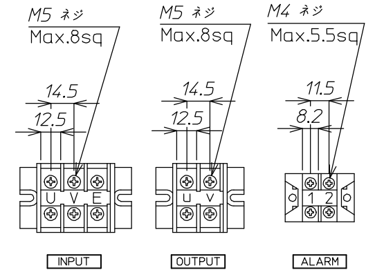
端子台詳細
