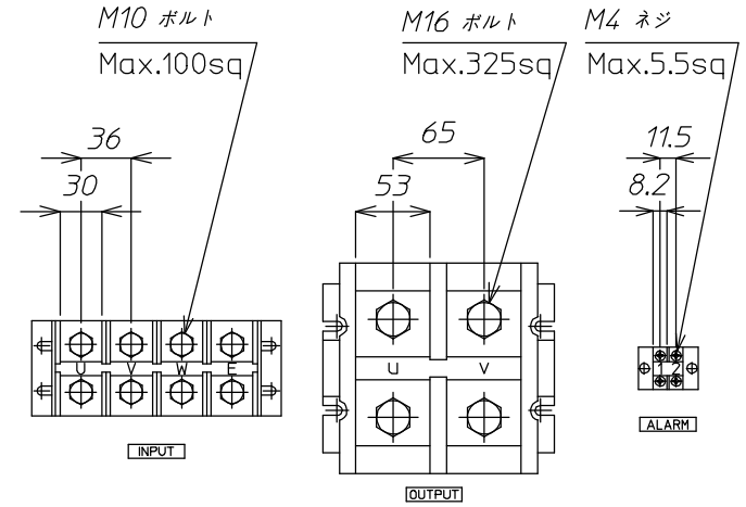
端子台詳細
