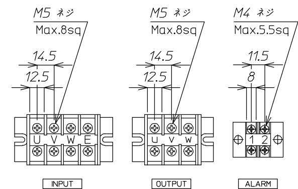
端子台詳細
